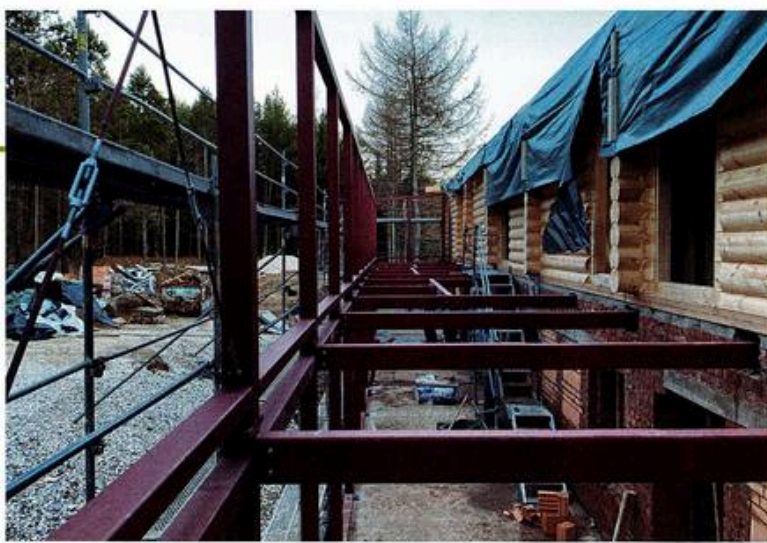
Für den Glasanbau sowie für den Zugang vom Jens-Weißflog-Hotel hat Peter Riedel Stahlkonstruktionen gefertigt.
